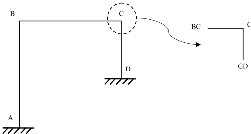
รูปที่ 1.10 จุดต่อแบบยึดรั้ง (Rigid Joint)
