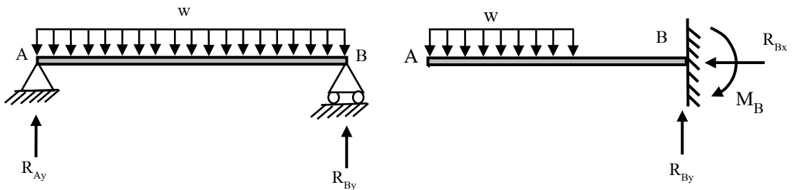
รูปที่ 1.4 ลักษณะของน้ำหนักกระทำแบบแผ่กระจายสม่ำเสมอ (Uniform Load)
