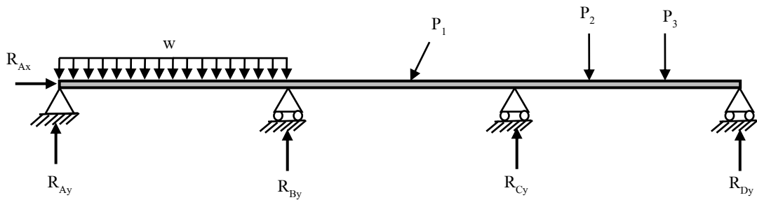
รูปที่ 1.18 (ต่อ) โครงสร้างแบบยาก (Indeterminate Structure)
