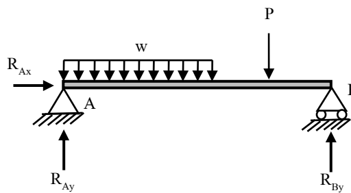
รูปที่ 1.19 โครงสร้างรับน้ำหนัก
