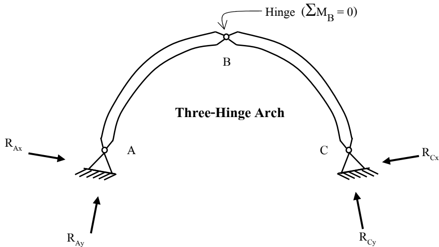
รูปที่ 1.16 โครงสร้างที่มีจำนวนของสมการสมดุลรวมกับสมการเงื่อนไขเท่ากับจำนวนตัวแปรไม่ทราบ
