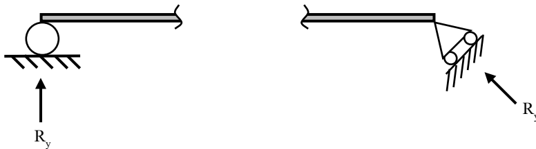
รูปที่ 1.6 สัญลักษณ์ของฐานรองรับแบบยึดหมุนเคลื่อนที่ได้ (Roller Support)
