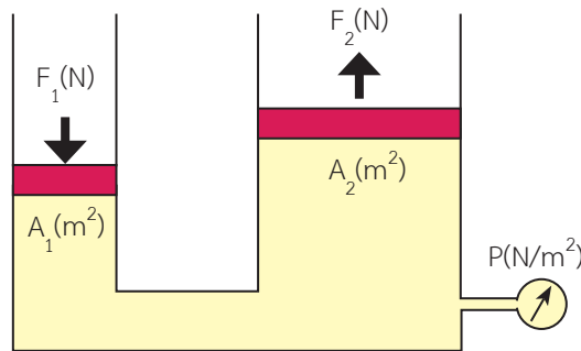
รูปที่ 1.4 แสดงกฎเบื้องต้นของลมอัด โดยแบลส์ ปาสคาล
